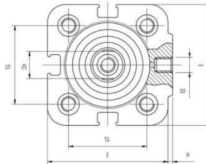
Ø 12-16-20-25
