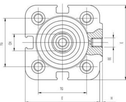
Ø 12-16-20-25
