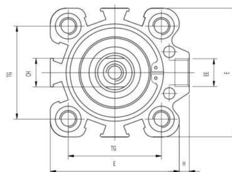
Ø 32-40-50-63-80-100
