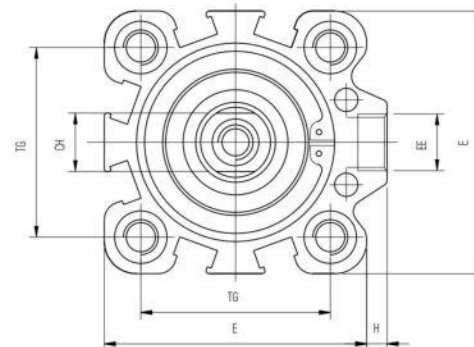
Ø 32-40-50-63-80-100
