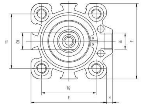
Ø 32-40-50-63-80-100
