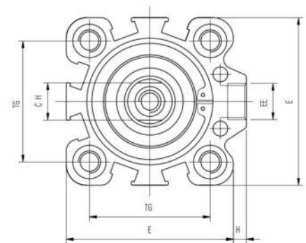
Ø 32-40-50-63-80-100
