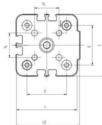
Ø 32-40-50-63-80-100
