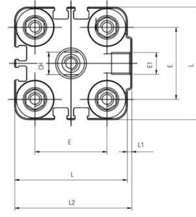
Ø 32-40-50-63-80-100
