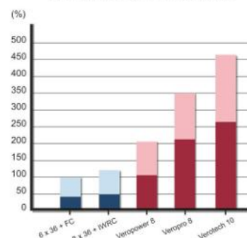
NÚMERO DE FLEXIONES ANTES DE DESCARTE Y ROTURA
