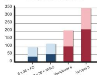
NÚMERO DE FLEXIONES ANTES DE DESCARTE Y ROTURA
