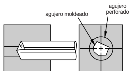
agujeros moldeados
