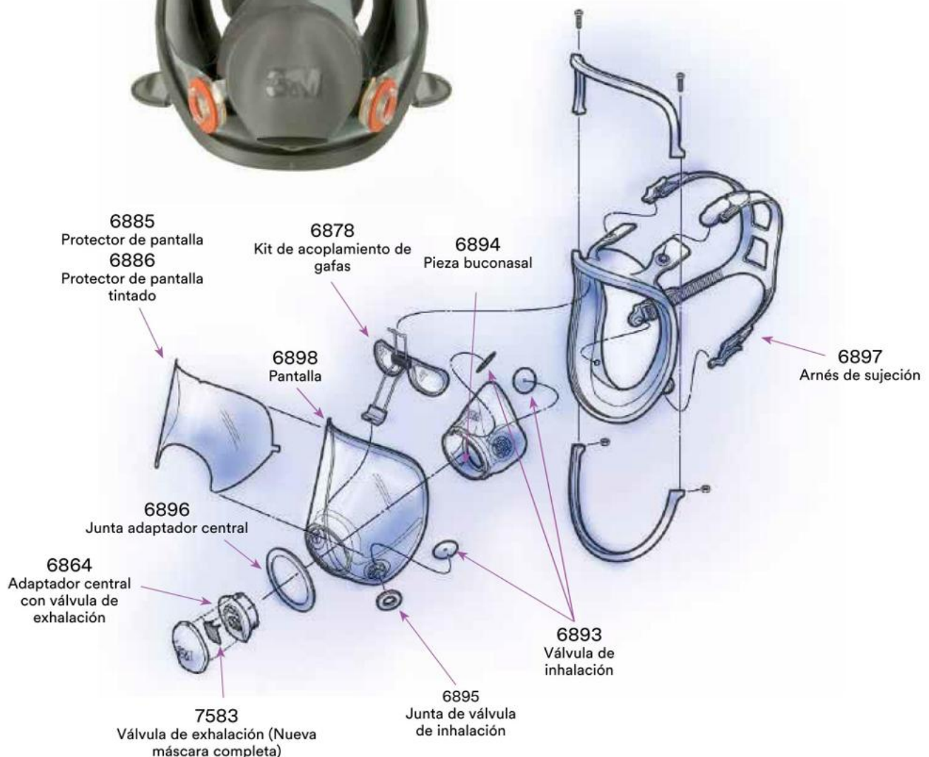
Despiece de Máscara Completa 3M Serie 6000: 6700S, 6800S y 6900S
